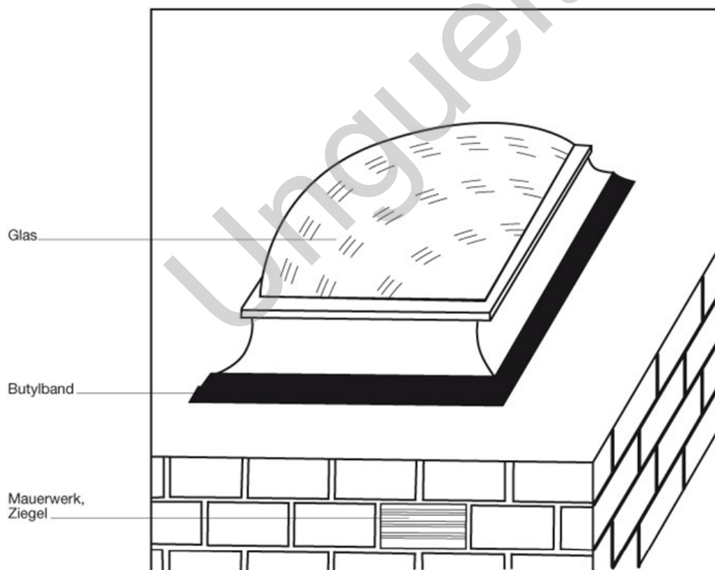
Abbildung 14: Lichtkuppelanschluss (Reparatur)
