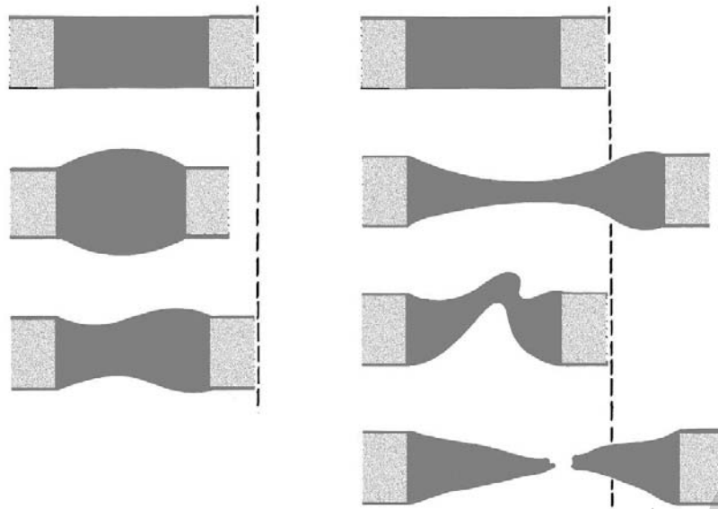
gestaucht Abbildung 23: Plastisches Verhalten
