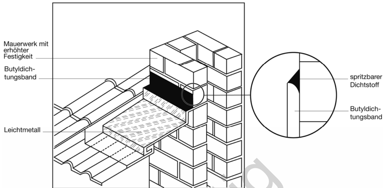
Abbildung 15: Kaminverwahrung (Reparatur)
