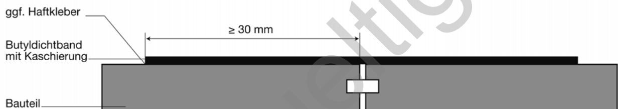
Abbildung 19 Verlegung flach
