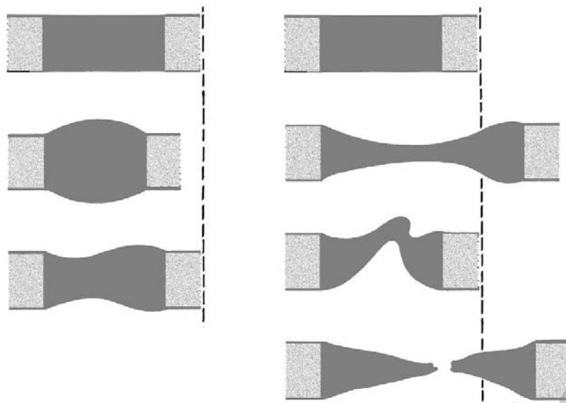
Abbildung 23: Plastisches Verhalten
