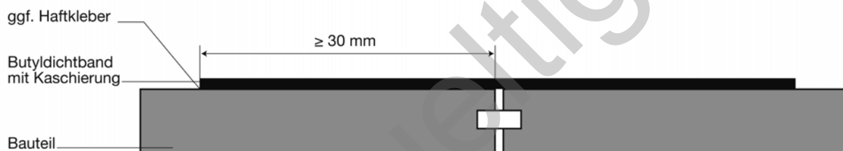
Abbildung 19 Verlegung flach
