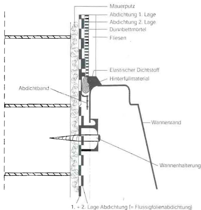
Abbildung 5: Anwendungsbeispiel für Wannenanschlussfugen
