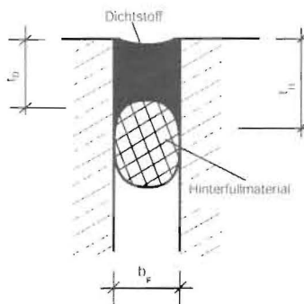
Abb. 1 Rechtecksfuge t_H = Tiefe der Haftfläche des Dichtstoffes t_D = Tiefe des Dichtstoffes b_F = Fugenbreite
