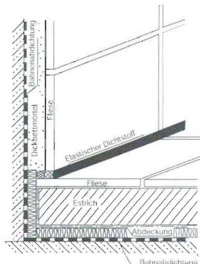
Abbildung 3: Boden-Wandanschlussfuge
