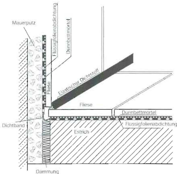
Abbildung 4: Randfuge als Dreiecksfuge
