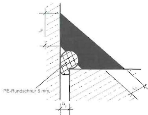
Abb. 2 Dreiecksfuge
