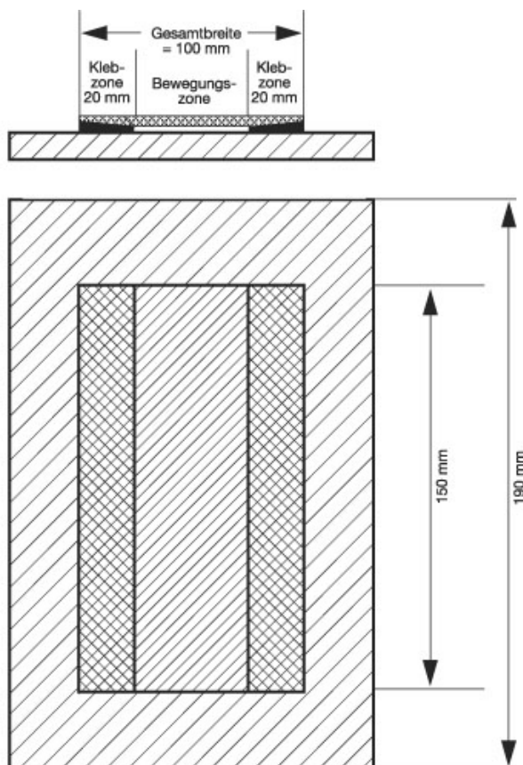
Bild 7: Probekörper; Prüfung nach Absatz 9.1 - Frühbeanspruchung -
