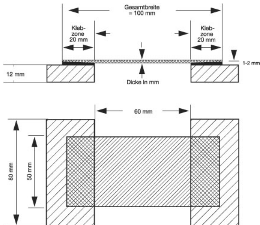
Bild 8: Probekörper; Prüfung nach Absatz 9.3 - Zugfestigkeit -
