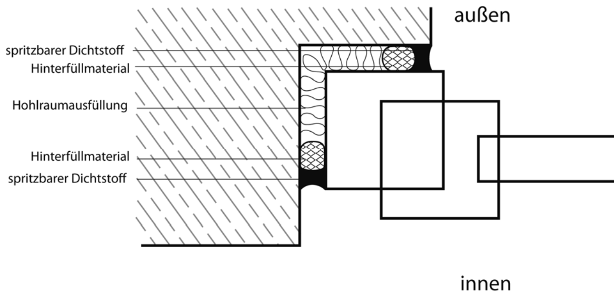
Bild 5: Fachgerechte Fugenausbildung beim Innenanslag
