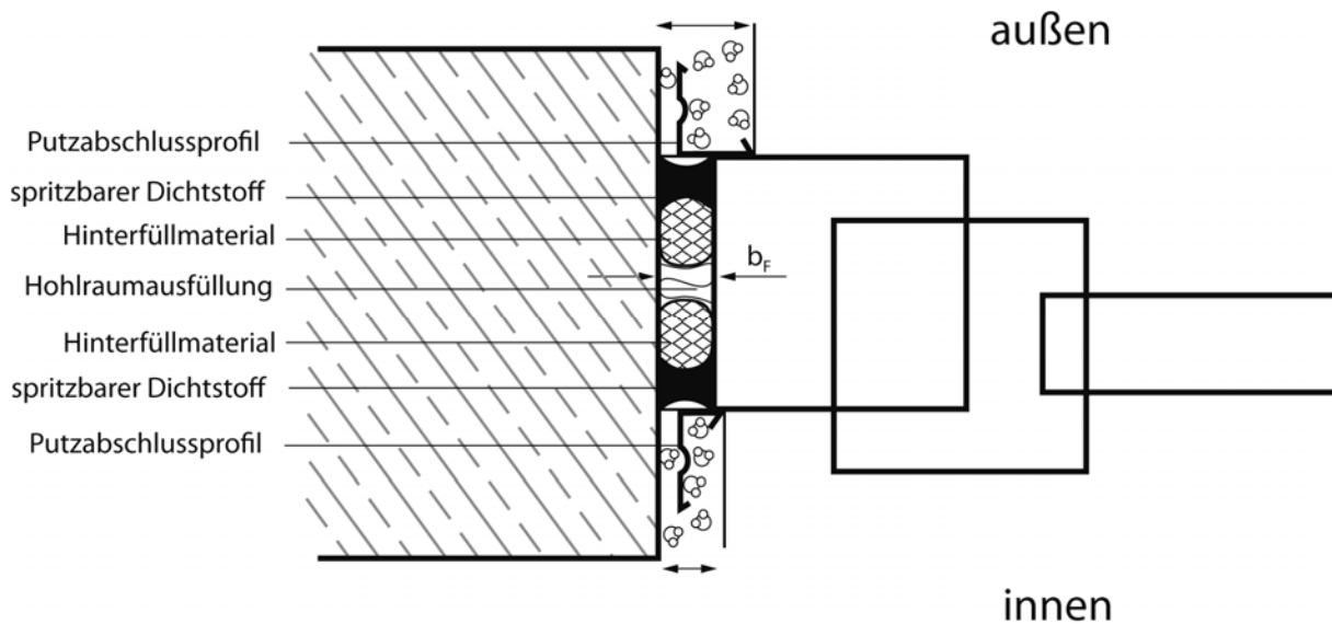
Bild 13.1: Fachgerechte Fugensanierung vor dem Verputzen des Baukörpers
